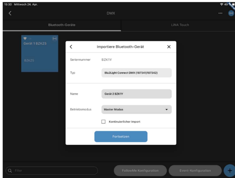
Abbildung 100: Modus Master
