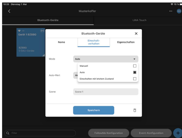
Abbildung 5: Auswahl Einschaltverhalten
