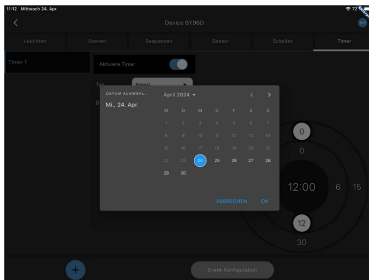
Abbildung 69: Einmaliger Timer
