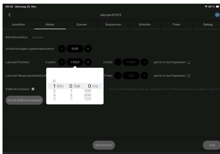
Abbildung 80: Modus Jalousie
