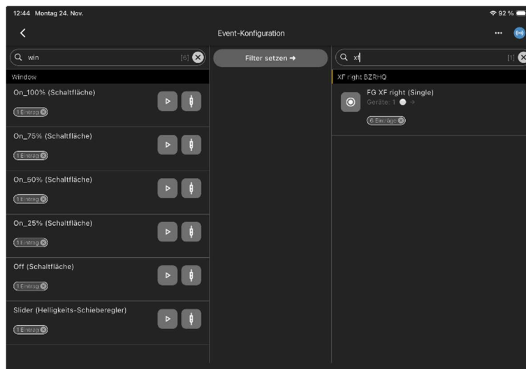
Abbildung 17: Event-Konfiguration
