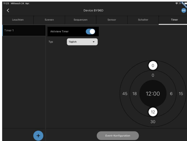
Abbildung 71: Täglicher Timer
