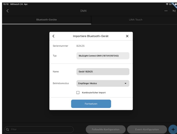
Abbildung 95: Modus Empfänger
