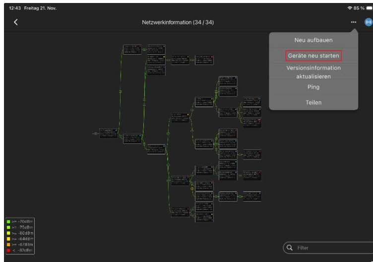
Abbildung 40: Netzwerkübersicht
