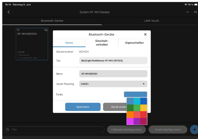
Abbildung 4: Farbauswahl
