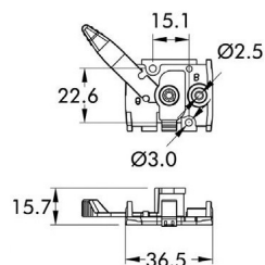
Держатель для track adapter № заказа: t.b.d.
