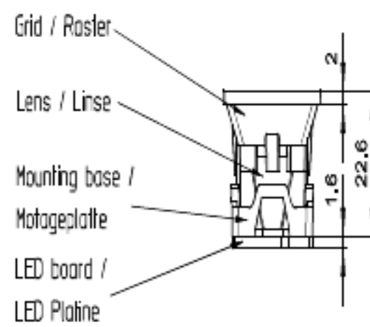
Assembly view / Zusammenbaudarstellung
