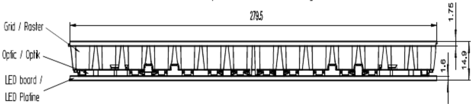
Assembly view / Zusammenbau darstellung
