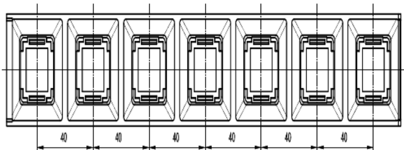
Assembly view / Zusammenbaudarstellung
